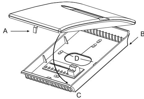
Fig. 10 EE245 enclosure
