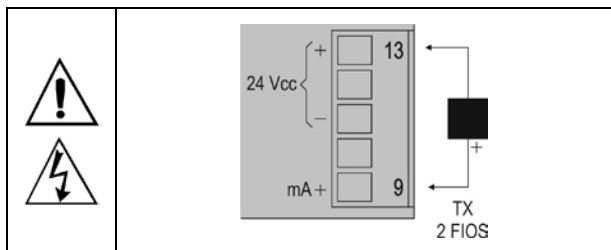
Figura 04 – Ejemplo de utilización de la fuente de tensión auxiliar del indicador
