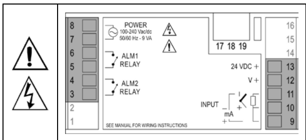
Figura 01 – Panel trasero del indicador
